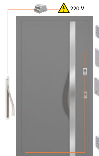
Fingerprint bei einer Alu Haustür im Flügel integriert inkl. Automatikschloss AV 4, Motoröffner, Netzteil, Kabelübergang und Fingerprint
